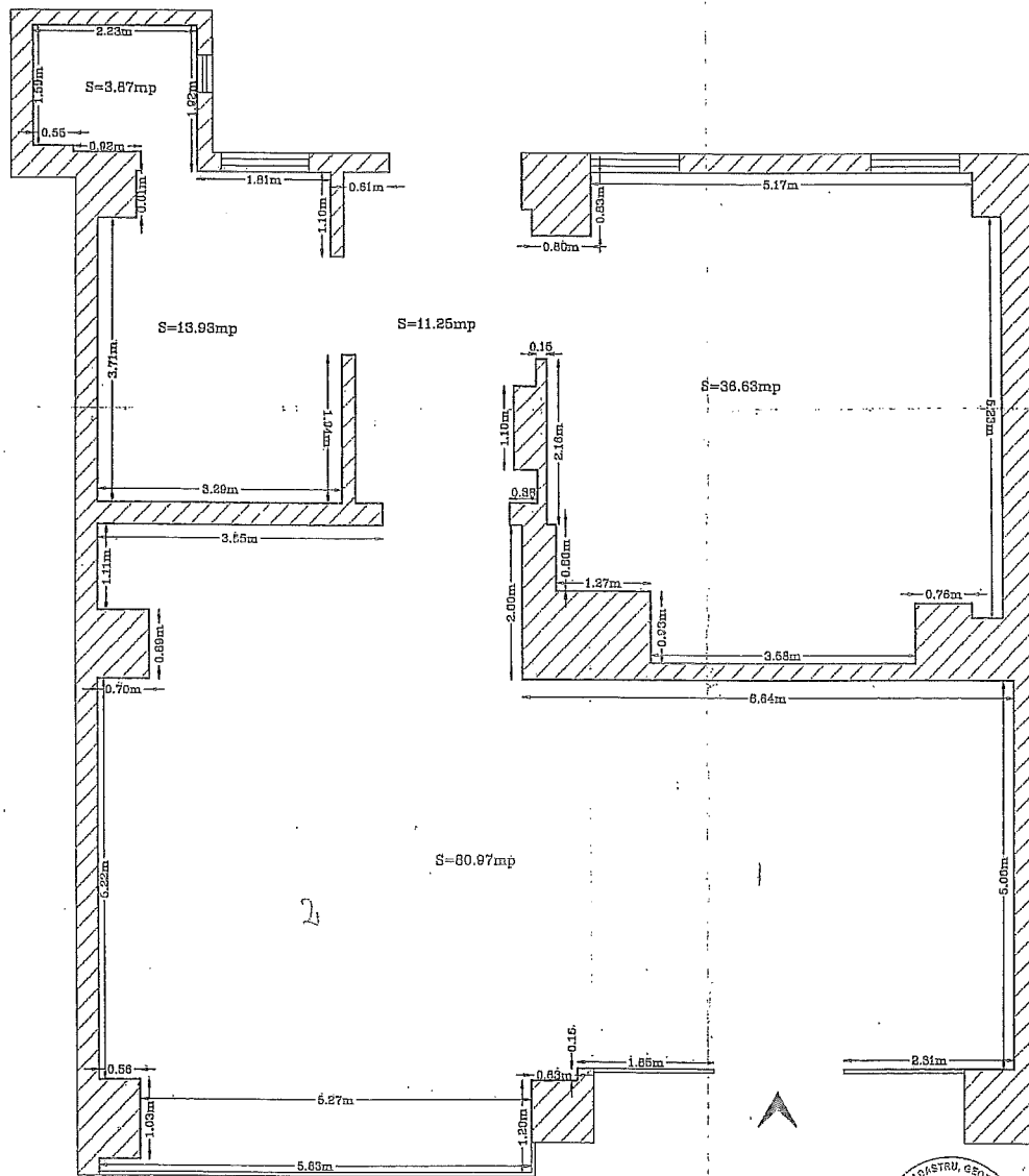
PLAN DE SITUATIE (RELEVU) Scara 1:50
